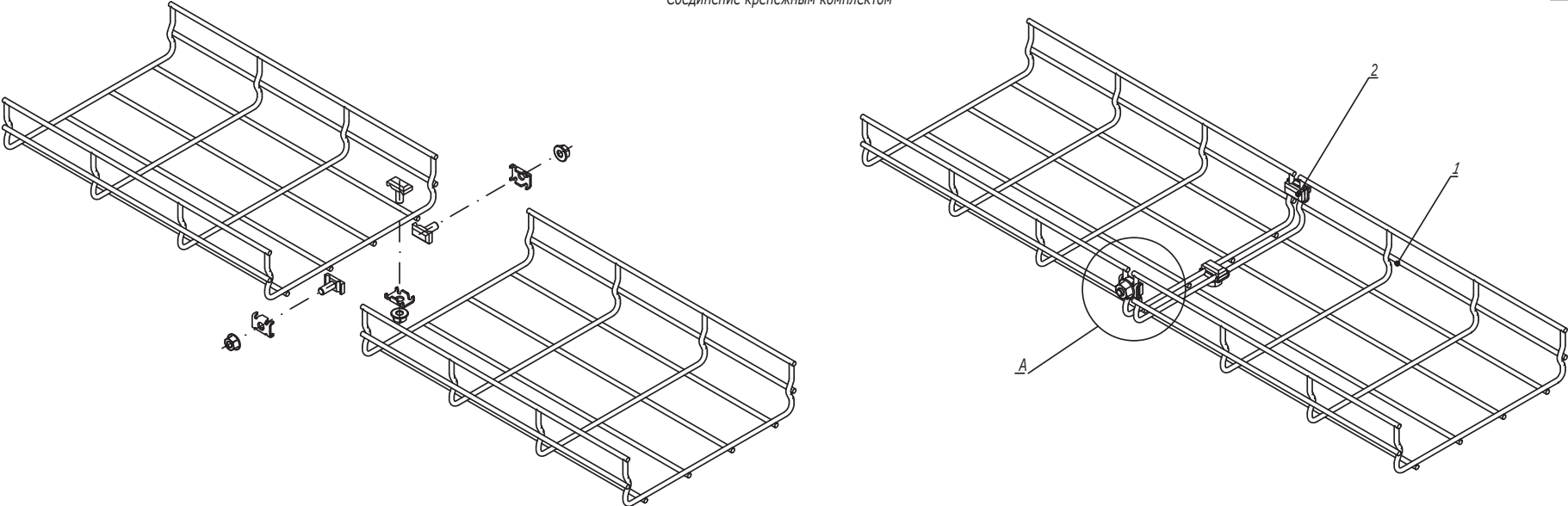
Соединение крепежным комплектом
