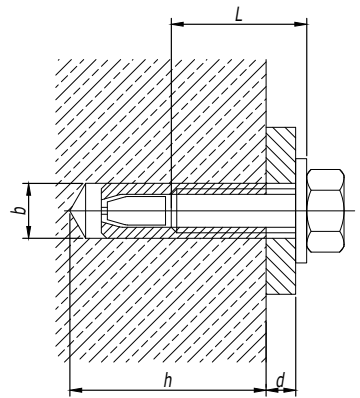
Стальной забивной анкер (тип 5)
