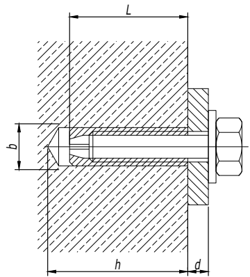
Латунный разрезной анкер (тип 6)
