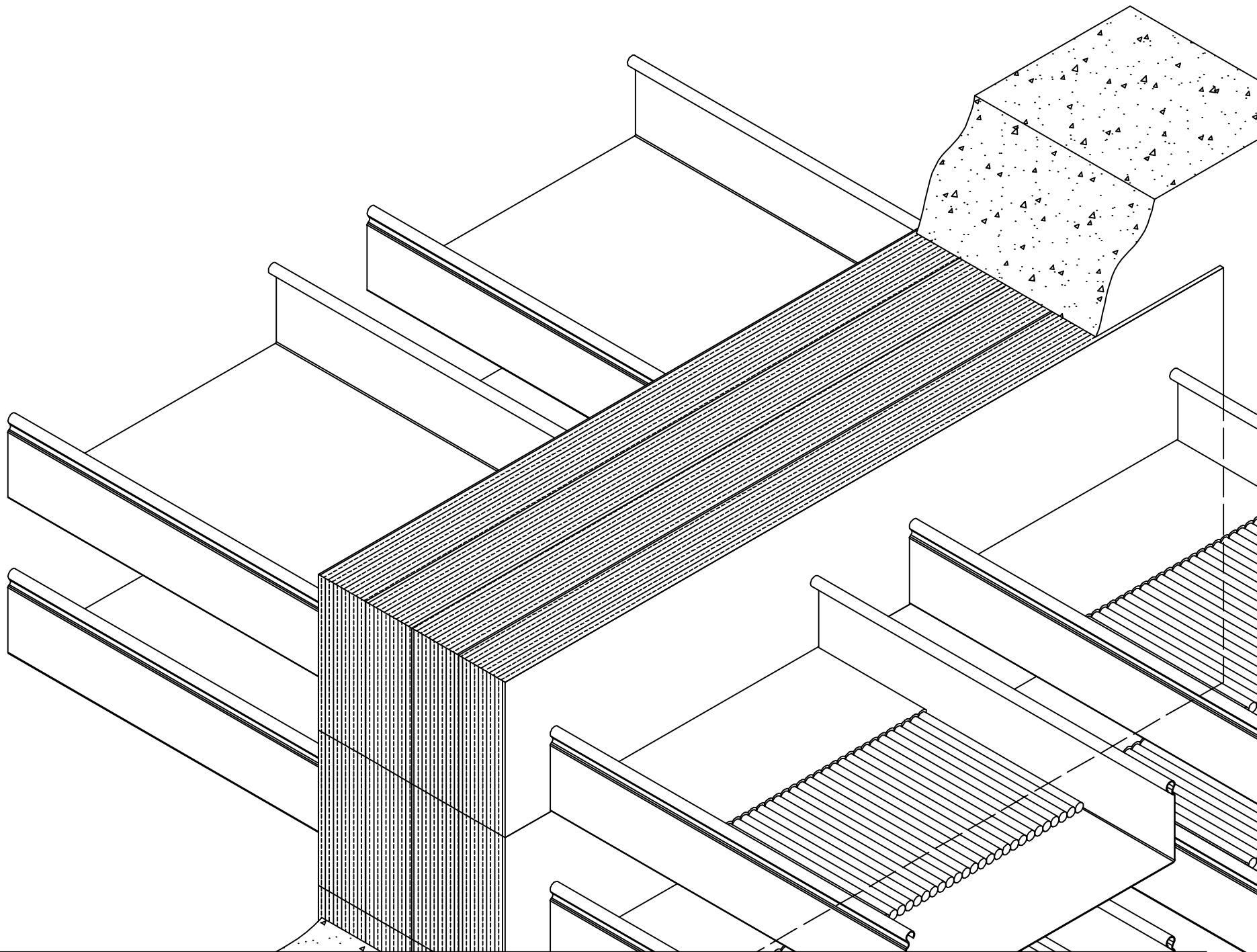
Пример организации прокладки группы лотков
